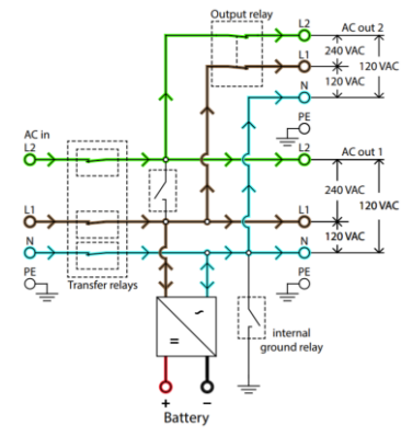
Flujo de energía, entrada de fase dividida
