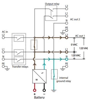
Flujo de energía: modo inversor
