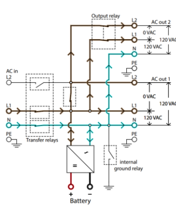
Flujo de energía, entrada de 120 V
